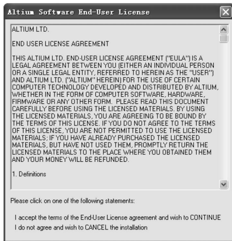
图 1-8 【协议】对话框
